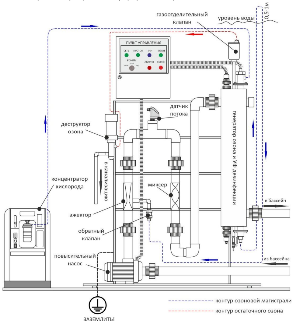
Схема компоновки устройств в составе системы
